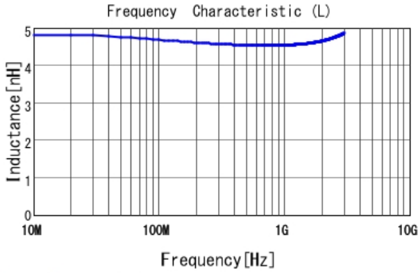
LQW04AN4N7C00 L
