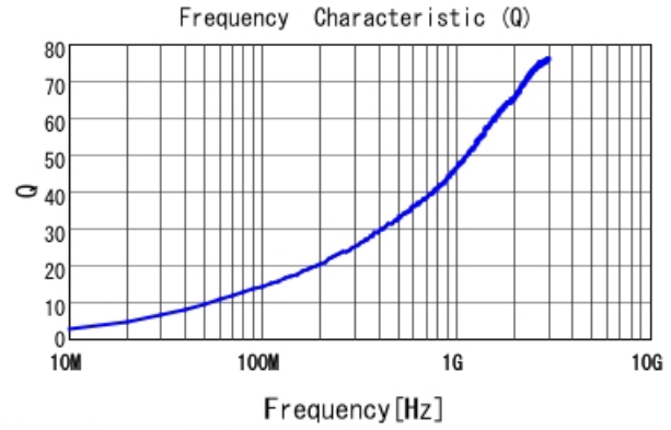
LQW04AN4N7C00 Q
