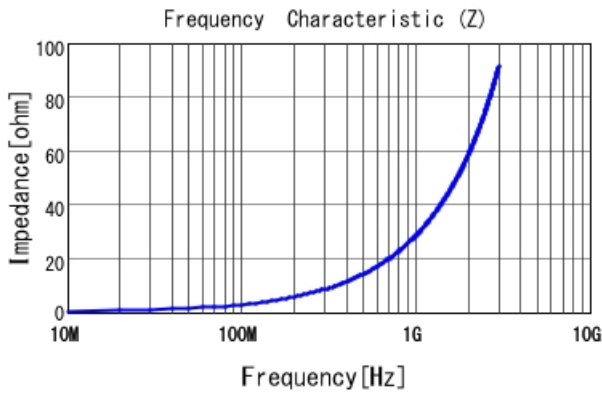
LQW04AN4N7C00 |Z|
