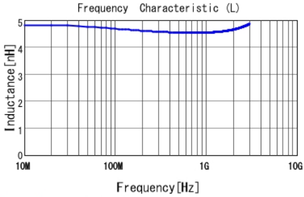
LQW04AN4N7D00 L
