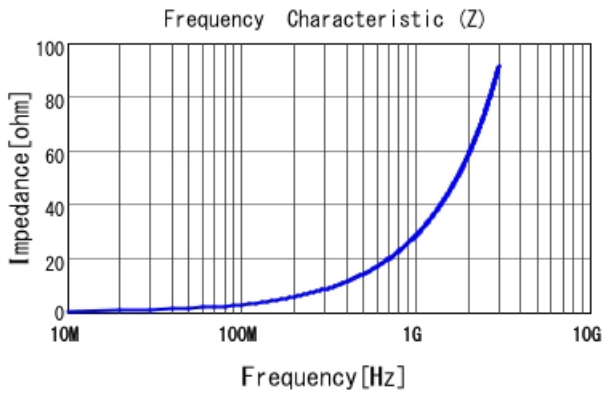
LQW04AN4N7D00 |Z|
