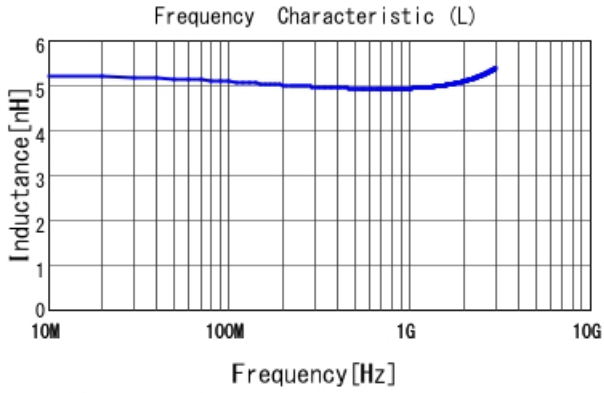
LQW04AN4N8D00 L
