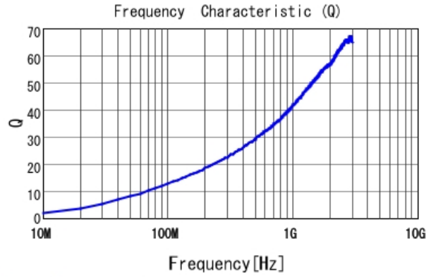
LQW04AN4N8D00 Q
