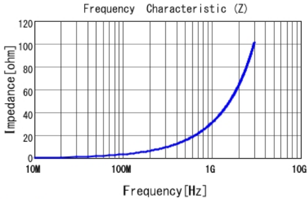
LQW04AN4N8D00 |Z|
