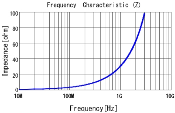
LQW04AN4N9C00 |Z|
