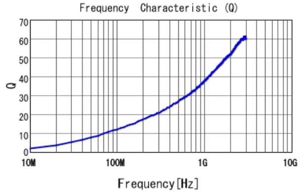
LQW04AN4N9C00 Q
