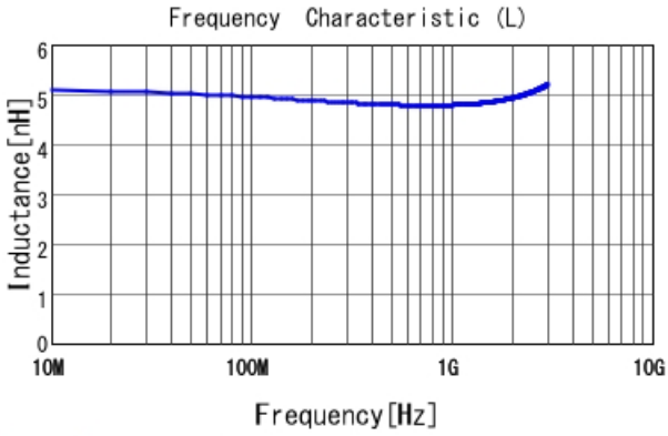
LQW04AN4N9C00 L
