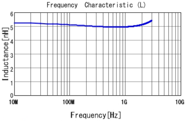
LQW04AN5N0C00 L
