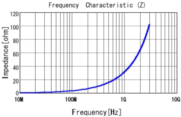
LQW04AN5N0C00 |Z|
