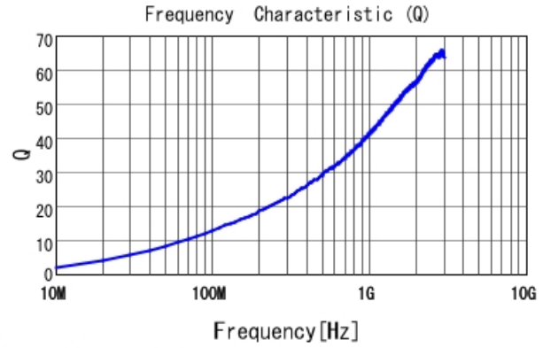
LQW04AN5N0C00 Q
