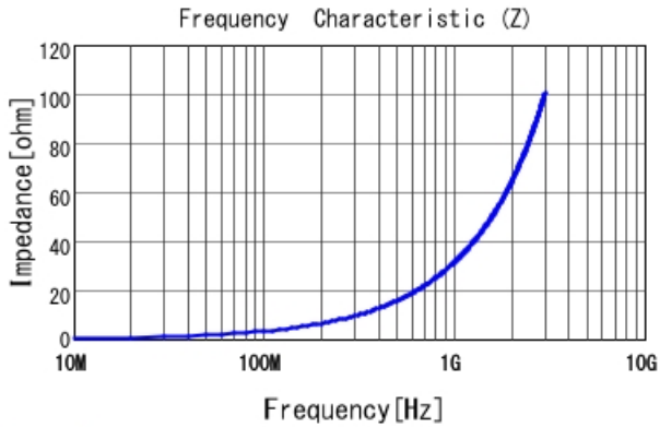
LQW04AN5N1C00 |Z|
