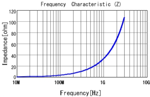
LQW04AN5N2C00 |Z|
