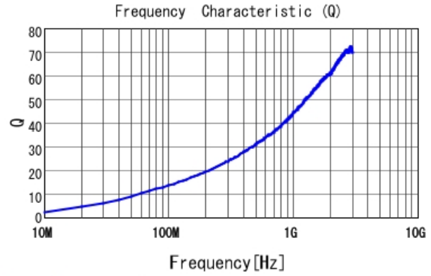
LQW04AN5N2C00 Q
