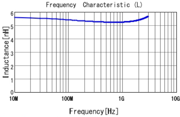
LQW04AN5N2C00 L
