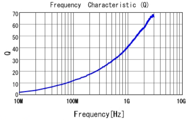
LQW04AN5N3D00 Q
