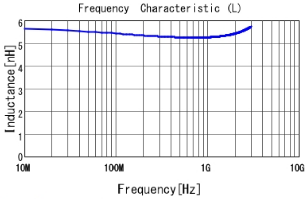
LQW04AN5N3D00 L
