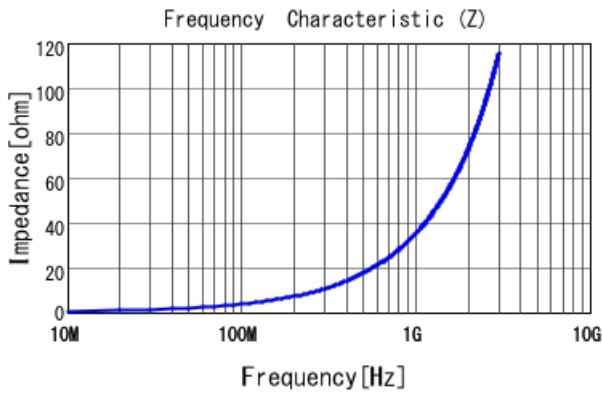
LQW04AN5N6C00 |Z|
