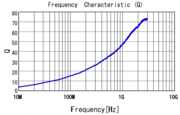
LQW04AN5N6C00 Q
