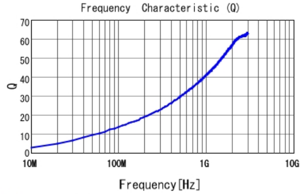
■ LQW04AN5N8C00 Q
