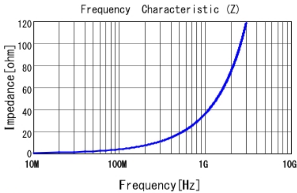
■ LQW04AN5N8C00 |Z|
