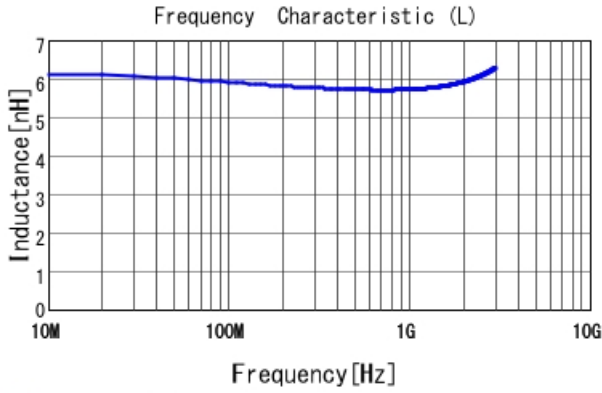
■ LQW04AN5N8C00 L
