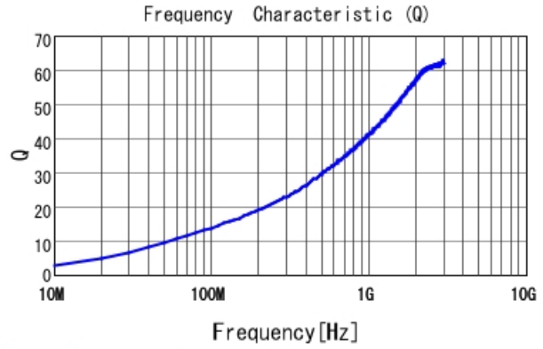
LQW04AN6N0C00 Q
