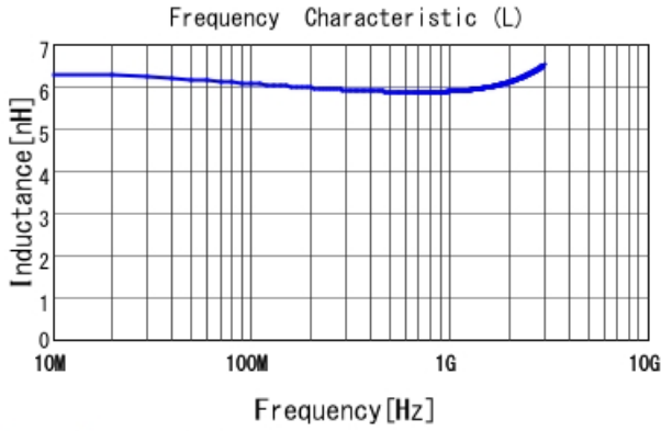
LQW04AN6N0C00 L
