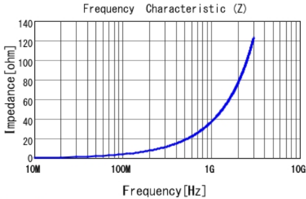
LQW04AN6N0C00 |Z|
