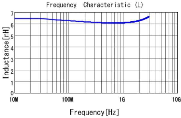
LQW04AN6N2C00 L
