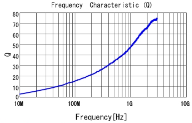
LQW04AN6N2C00 Q
