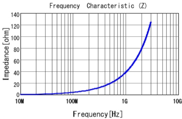
LQW04AN6N2C00 |Z|
