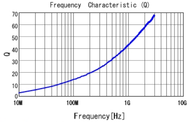
LQW04AN6N4D00 Q
