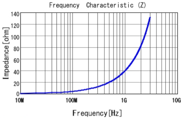
LQW04AN6N4D00 |Z|
