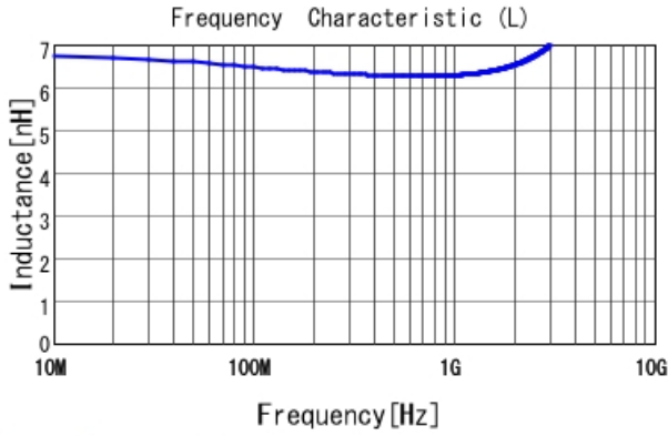
LQW04AN6N4D00 L
