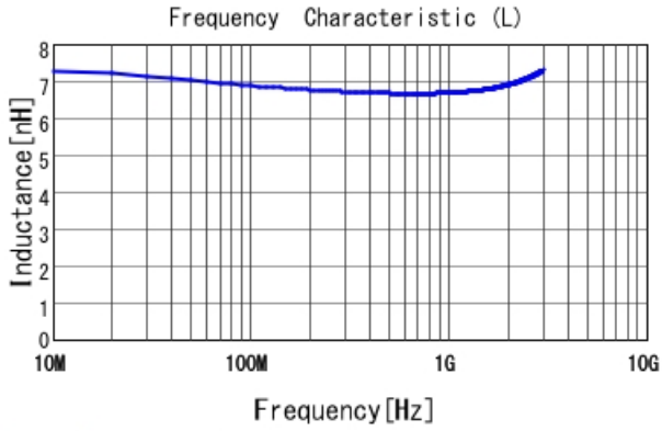
LQW04AN6N8C00 L
