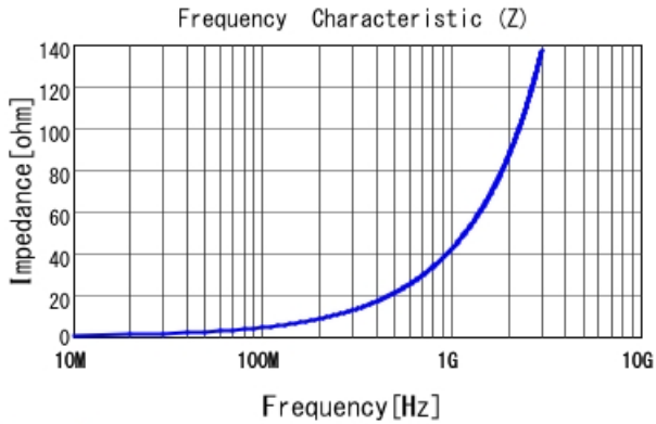
LQW04AN6N8C00 |Z|
