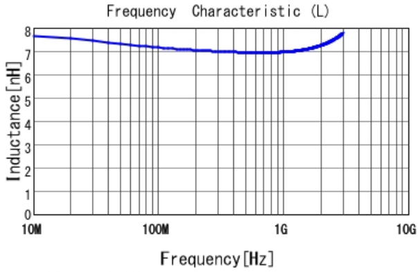
LQW04AN7N0D00 L
