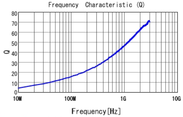
LQW04AN7N0D00 Q
