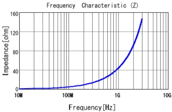
LQW04AN7N0D00 |Z|
