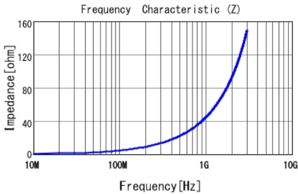
LQW04AN7N1C00 |Z|
