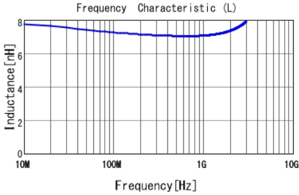
LQW04AN7N1C00 L
