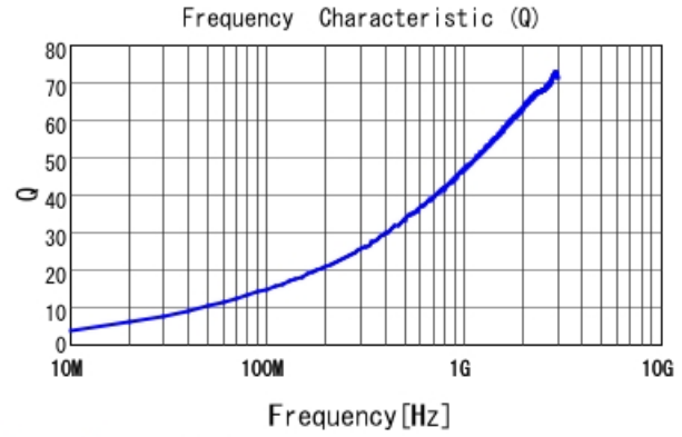
LQW04AN7N1C00 Q
