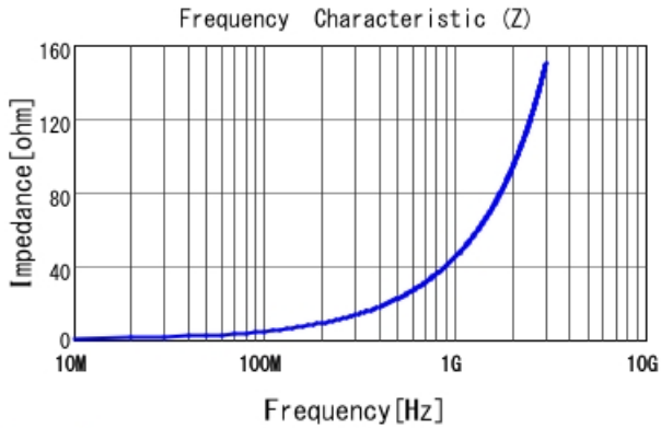
LQW04AN7N2C00 |Z|
