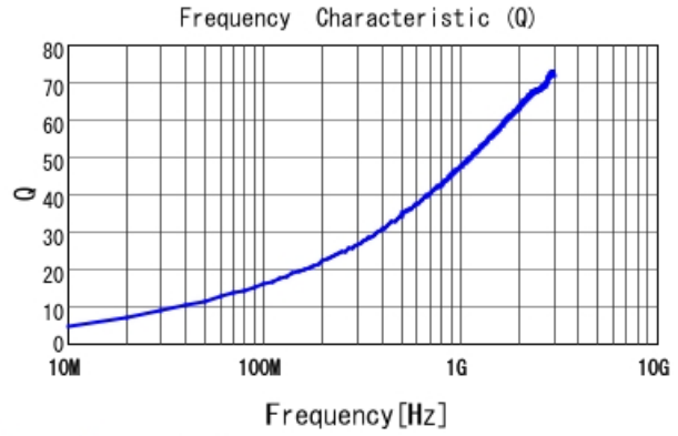
LQW04AN7N2C00 Q
