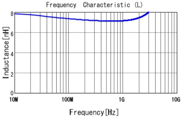
LQW04AN7N2C00 L
