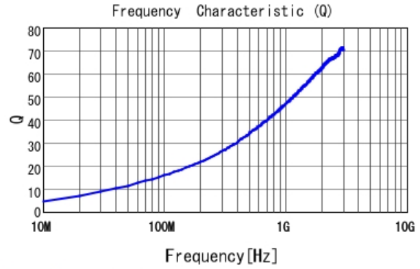
LQW04AN7N3D00 Q
