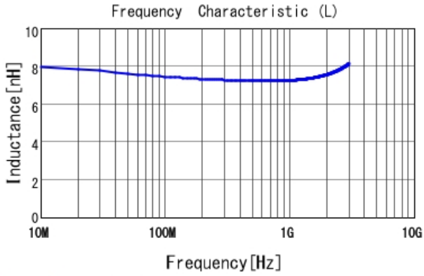
LQW04AN7N3D00 L
