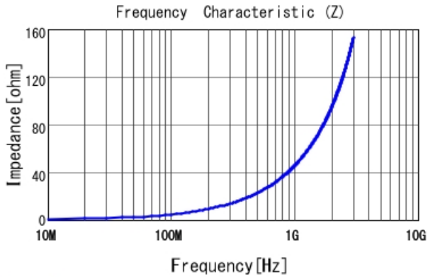
LQW04AN7N3D00 |Z|
