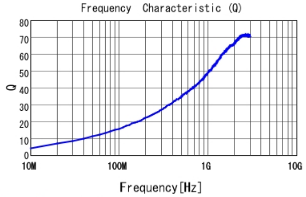
LQW04AN7N5D00 Q
