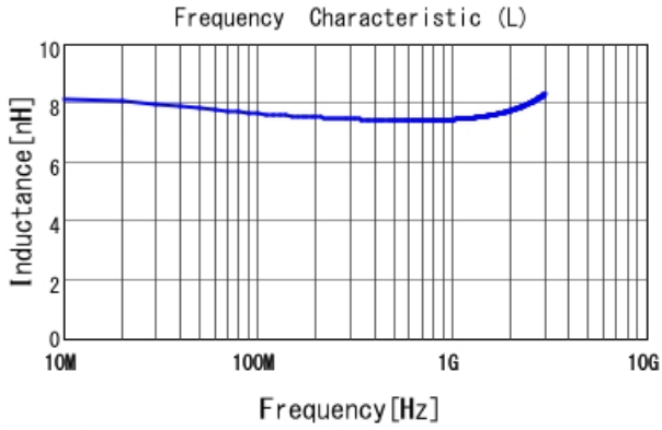
LQW04AN7N5D00 L
