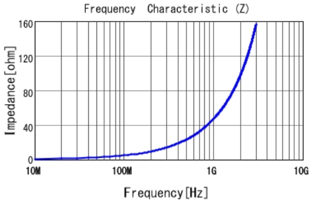
LQW04AN7N5D00 |Z|
