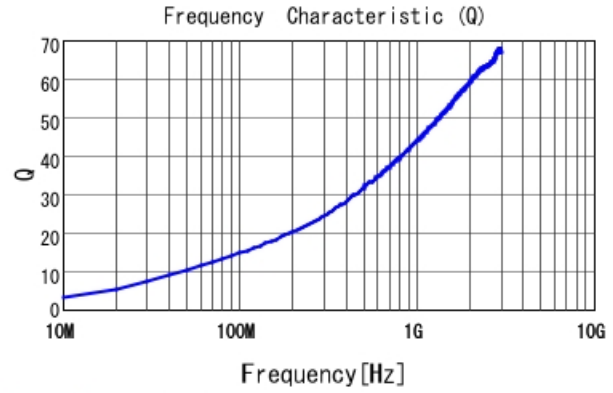
LQW04AN7N8D00 Q
