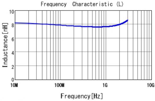
LQW04AN7N8D00 L
