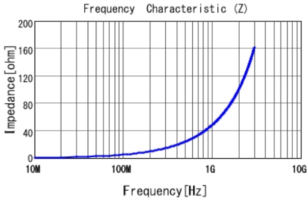
LQW04AN7N8D00 |Z|
