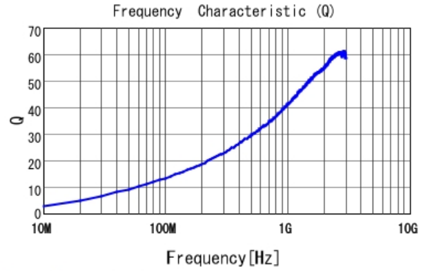
LQW04AN7N9C00 Q
