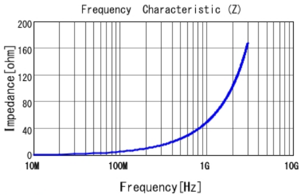
LQW04AN7N9C00 |Z|
