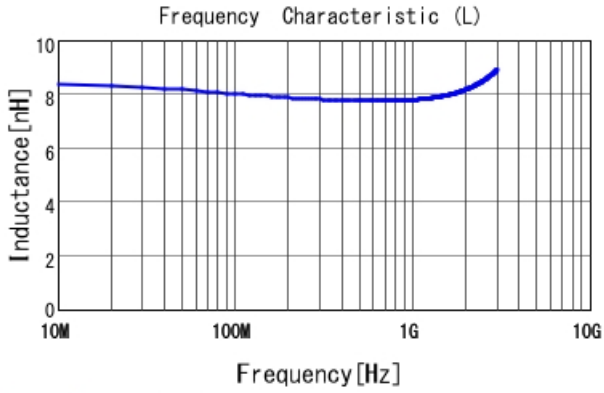
LQW04AN7N9C00 L
