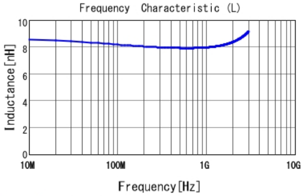
LQW04AN8N0C00 L
