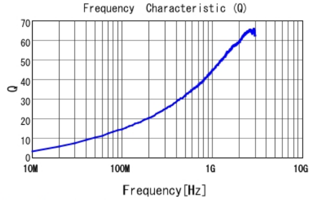
LQW04AN8N0C00 Q
