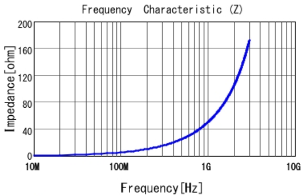
LQW04AN8N0C00 |Z|
