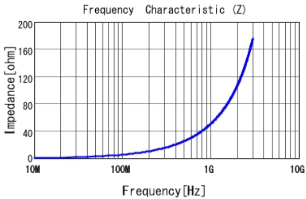
LQW04AN8N1C00 |Z|
