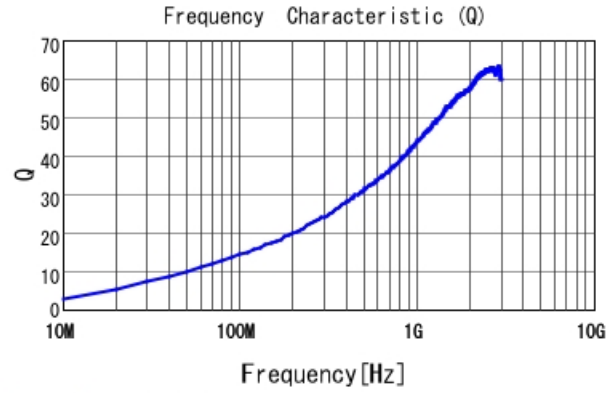
LQW04AN8N1D00 Q
