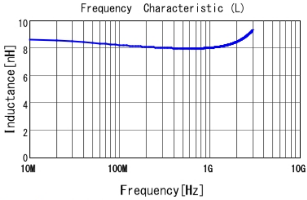
LQW04AN8N1D00 L
