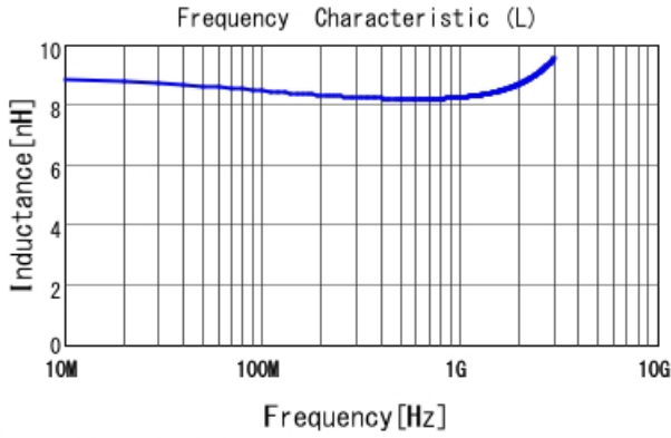
LQW04AN8N4D00 L
