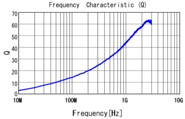
LQW04AN8N4D00 Q
