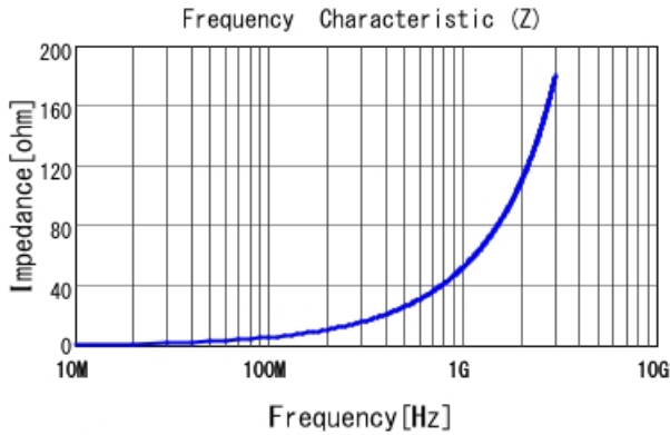
LQW04AN8N4D00 |Z|
