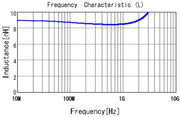
LQW04AN8N5C00 L
