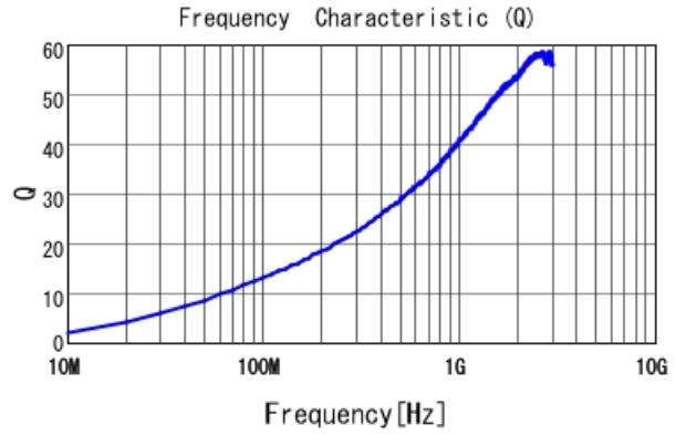
LQW04AN8N5C00 Q
