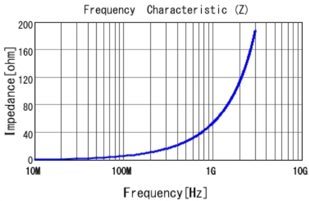
LQW04AN8N5C00 |Z|
