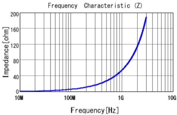
LQW04AN8N6C00 |Z|
