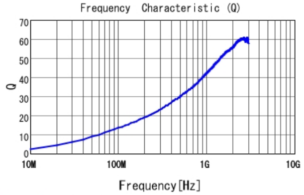
LQW04AN8N6C00 Q
