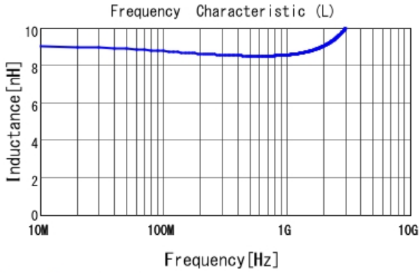
LQW04AN8N6C00 L
