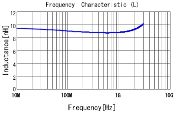
LQW04AN8N9D00 L
