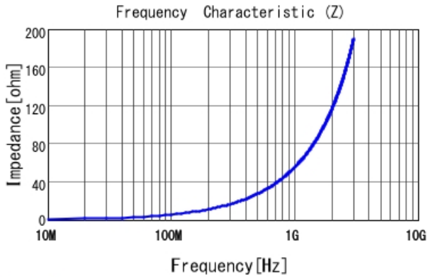
LQW04AN8N9D00 |Z|
