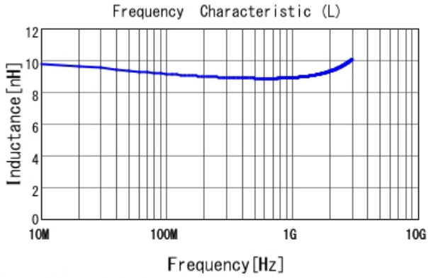
LQW04AN9N1D00 L
