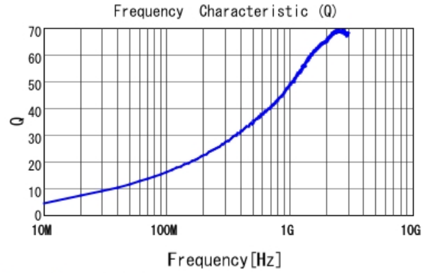
LQW04AN9N1D00 Q
