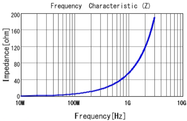
LQW04AN9N1D00 |Z|
