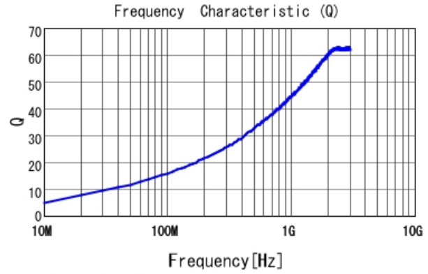
LQW04AN9N2C00 Q
