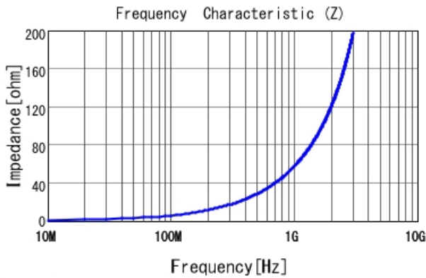
LQW04AN9N2C00 |Z|
