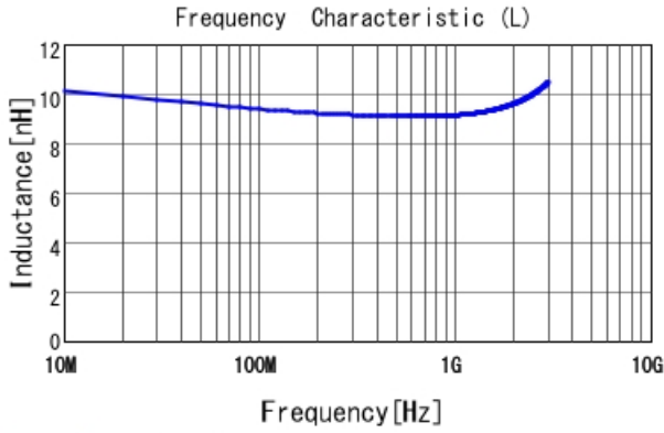
LQW04AN9N2C00 L
