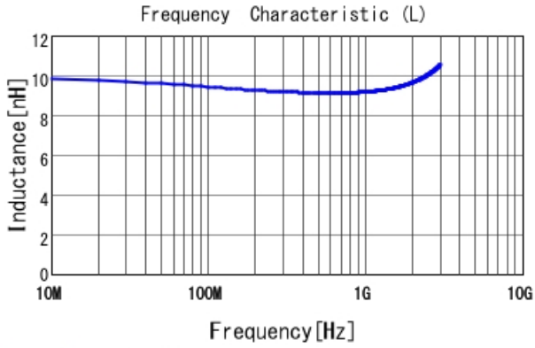
LQW04AN9N3C00 L
