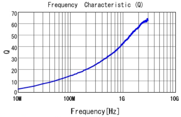
LQW04AN9N3C00 Q
