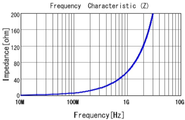
LQW04AN9N3C00 |Z|
