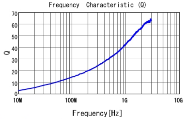
LQW04AN9N3D00 Q
