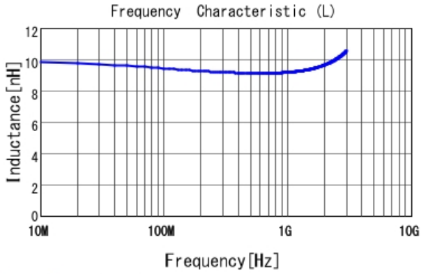
LQW04AN9N3D00 L
