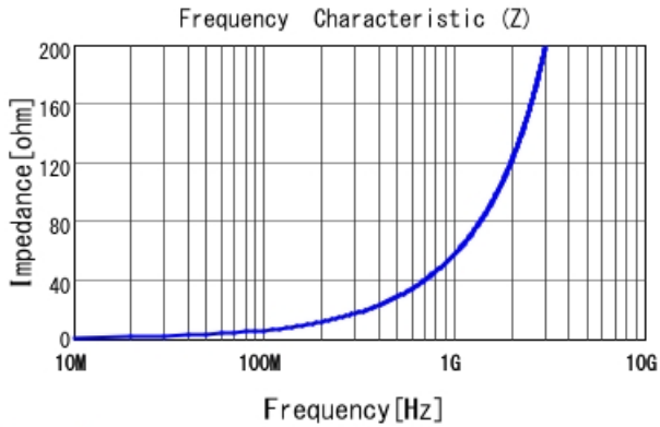
LQW04AN9N3D00 |Z|
