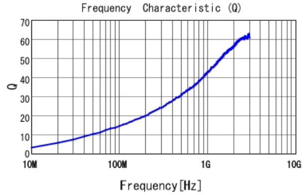
LQW04AN9N4D00 Q
