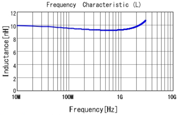
LQW04AN9N4D00 L
