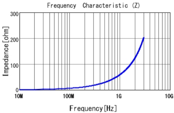
LQW04AN9N5D00 |Z|
