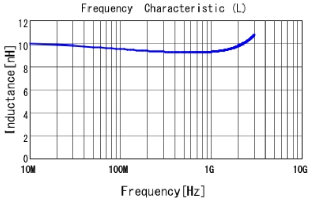
LQW04AN9N5D00 L
