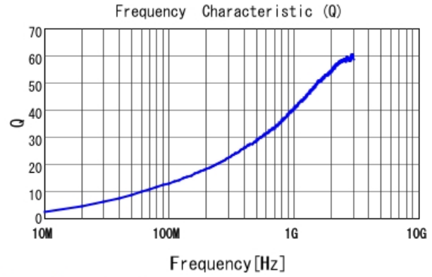
LQW04AN9N5D00 Q
