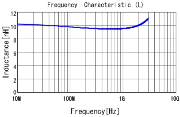
LQW04AN9N7C00 L
