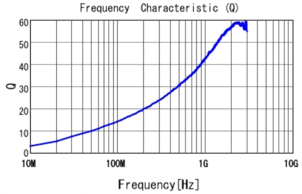
LQW04AN9N7C00 Q
