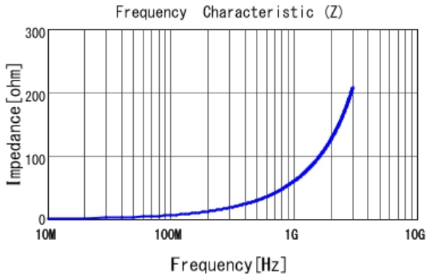
LQW04AN9N7C00 |Z|
