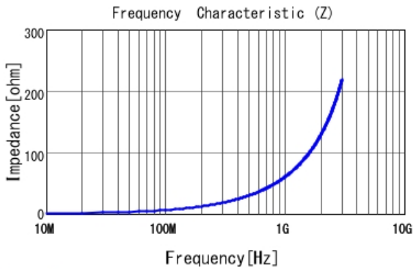
LQW04AN9N8C00 |Z|
