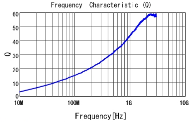
LQW04AN9N8C00 Q
