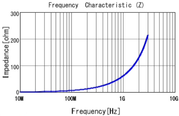
LQW04AN9N9C00 |Z|
