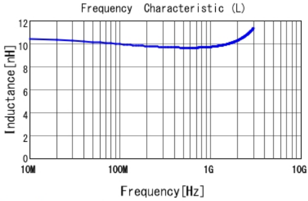
LQW04AN9N9C00 L
