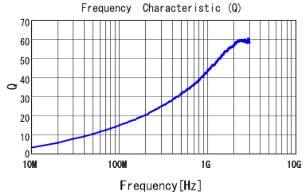
LQW04AN9N9C00 Q
