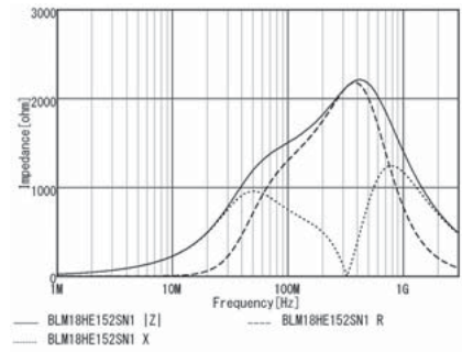
BLM18HE152SN1
