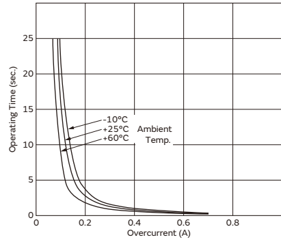
PTGL05AR181M9N51B0
