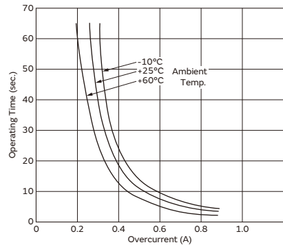
PTGL09AR250H8B52B0
