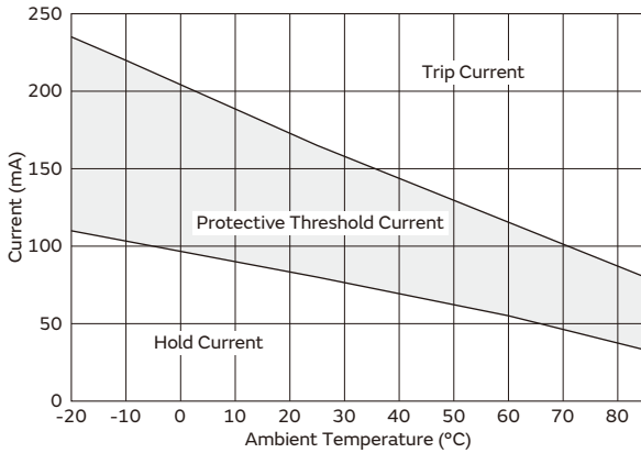
PRG18BC100MM1RB
