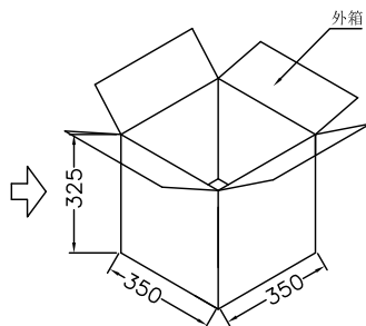
外箱
