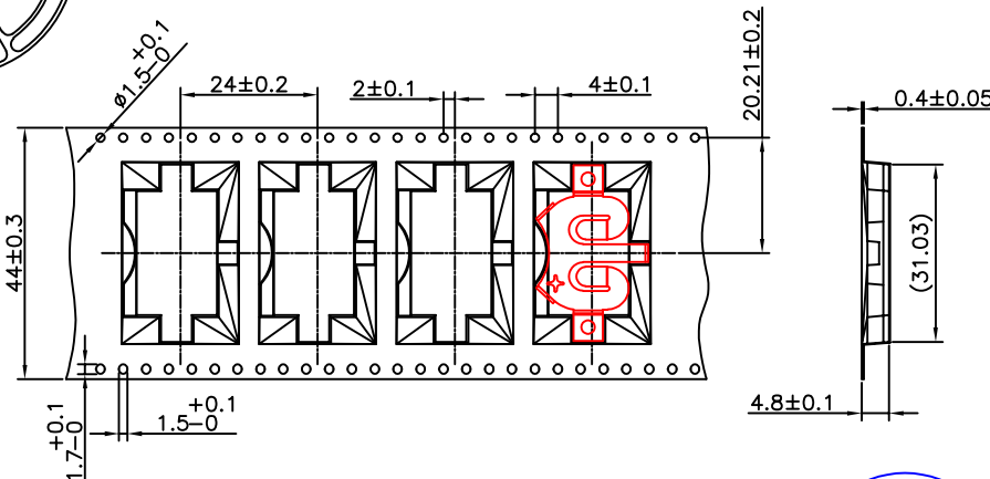
工程图
