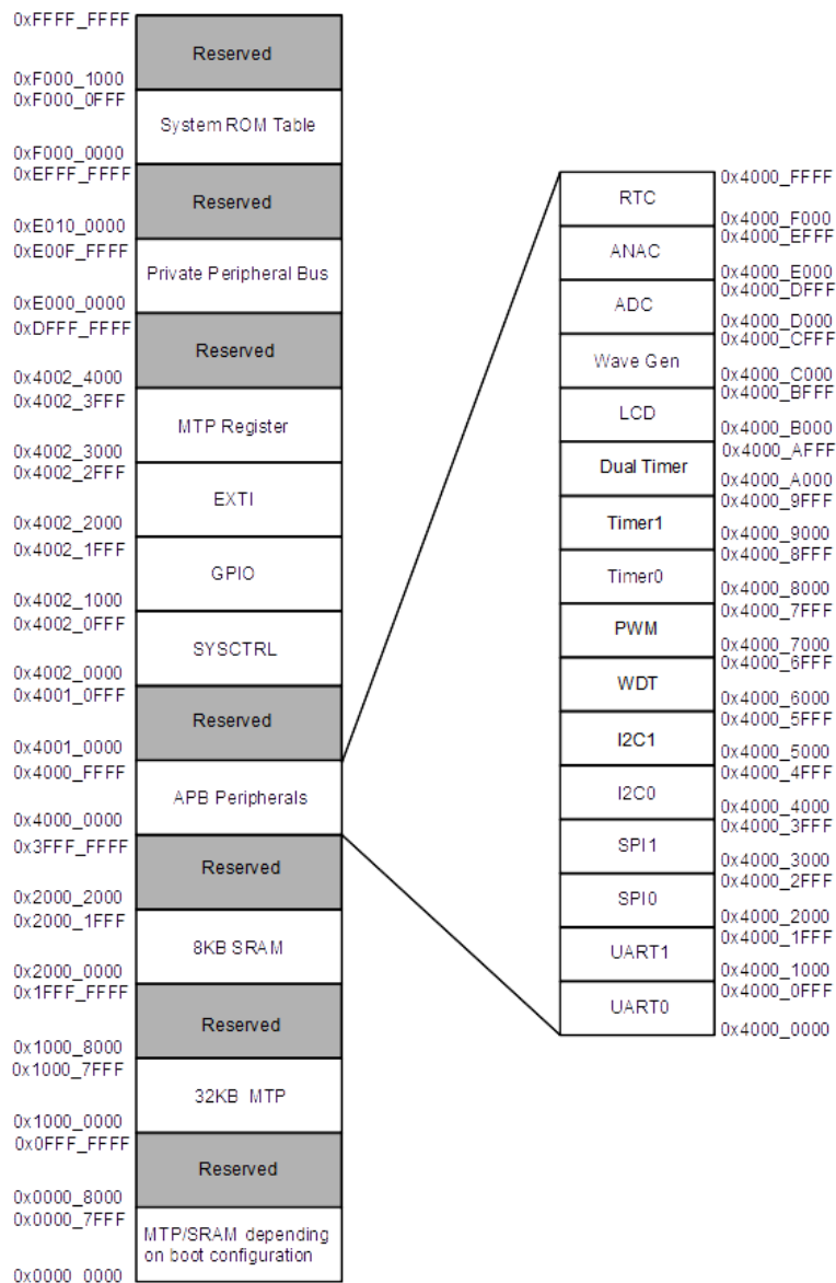
图 5 内存映射图
