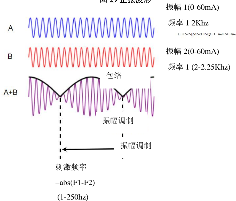
图 29 正弦波形
