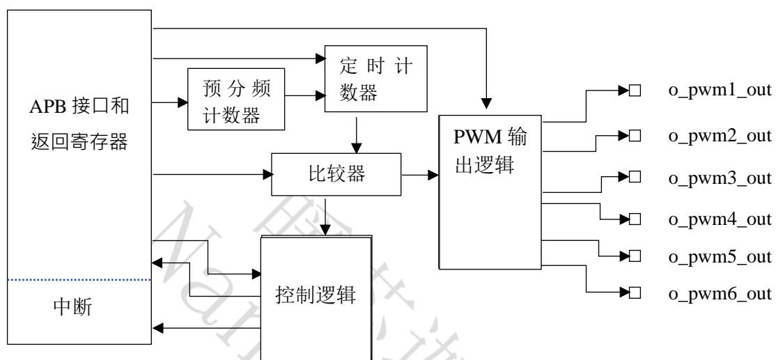
图 23 PWM 框图
