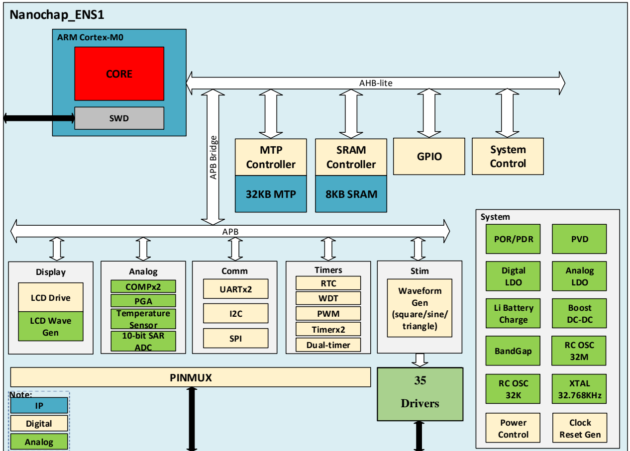
图 1 原理框图
