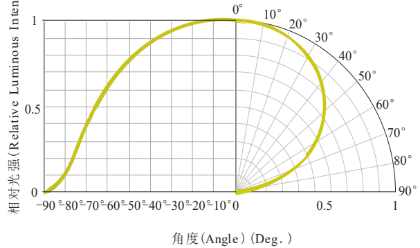
光强分布特性曲线 Typical Spatial Distribution
