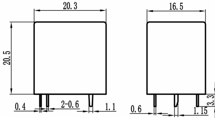
外形尺寸图
