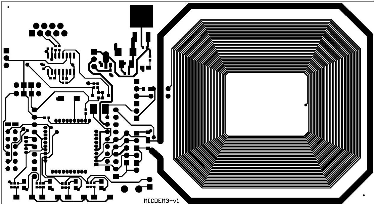
„Bottom” layer
