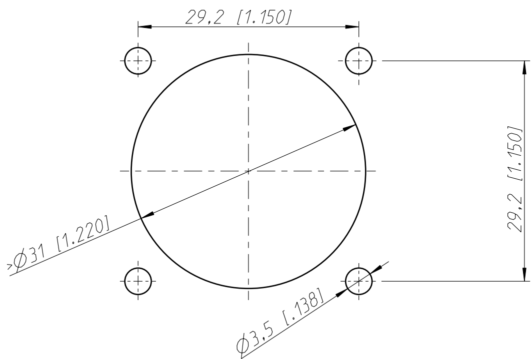
Panel Cut Out (Frontplattenausschnitt)
