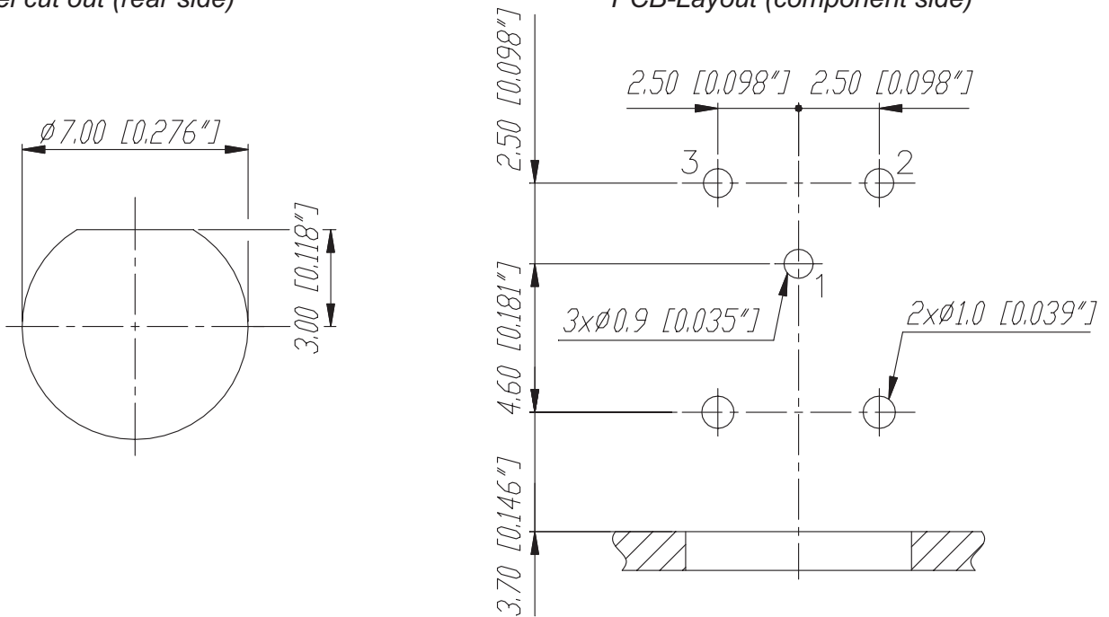
Frontplattenausschnitt (Rückseite) Panel cut out (rear side)
