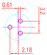
3-POLE:
