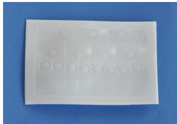
型号: 7703-1 尺寸: 60.6*42.4 焦距: 30.5mm 感应角度: 83 ° 感应距离: 24m
