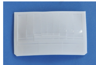
型号: SIR 650P 尺寸: 59.4*38.9 焦距: 30mm 感应角度: 120。 感应距离: 12m
