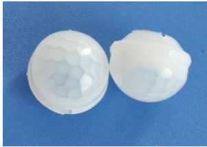
型号: 018090 尺寸: \varnothing 17.9 \times 13.9 焦距: 9mm 感应角度: 120° 感应距离: 8m
