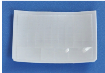
型号: SIR-650 尺寸: 59.5*38.9 焦距: 30mm 感应角度: 120 ° 感应距离: 12m
