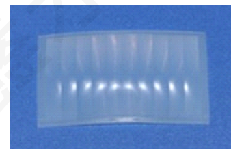
型号: 8719-A 尺寸: 53.5*31 焦距: 25mm 感应角度: 100° 感应距离: 10-11m
