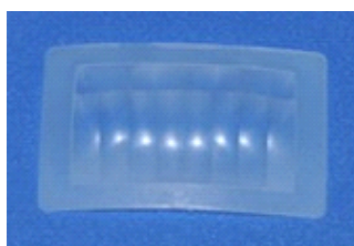
型号: 7803-1 尺寸: 39*25 焦距: 20mm 感应角度: 89° 感应距离: 7m
