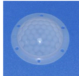
型号: 4/1 球 尺寸: 52.6*31*23.1*29 焦距: 30mm 感应角度: 100° 感应距离: 10m
